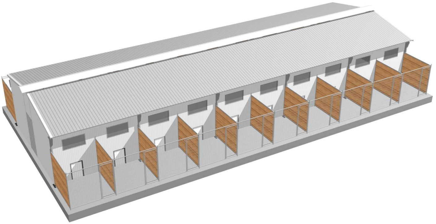
ΕΙΚΟΝΑ 7 : ΠΛΑΪΝΗ ΕΙΚΟΝΑ ΚΑΤΑΦΥΓΙΟΥ
