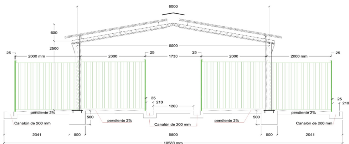
ΕΙΚΟΝΑ 5: ΕΝΔΕΙΚΤΙΚΗ ΤΟΜΗ ΚΑΤΑΦΥΓΙΟΥ
