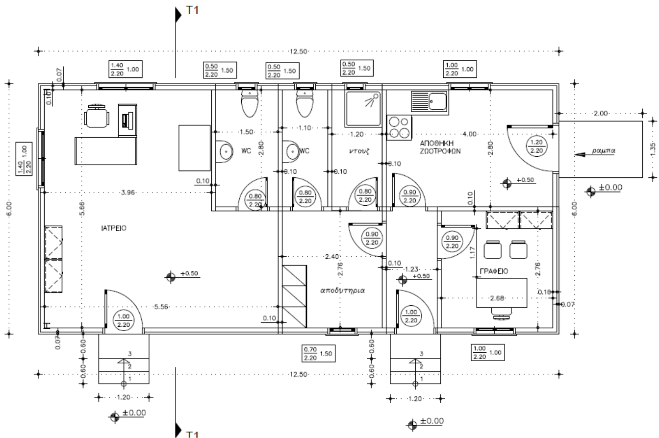
ΕΙΚΟΝΑ 11 : ΚΑΤΟΨΗ ΚΤΗΡΙΟΥ ΔΙΟΙΚΗΣΗΣ
